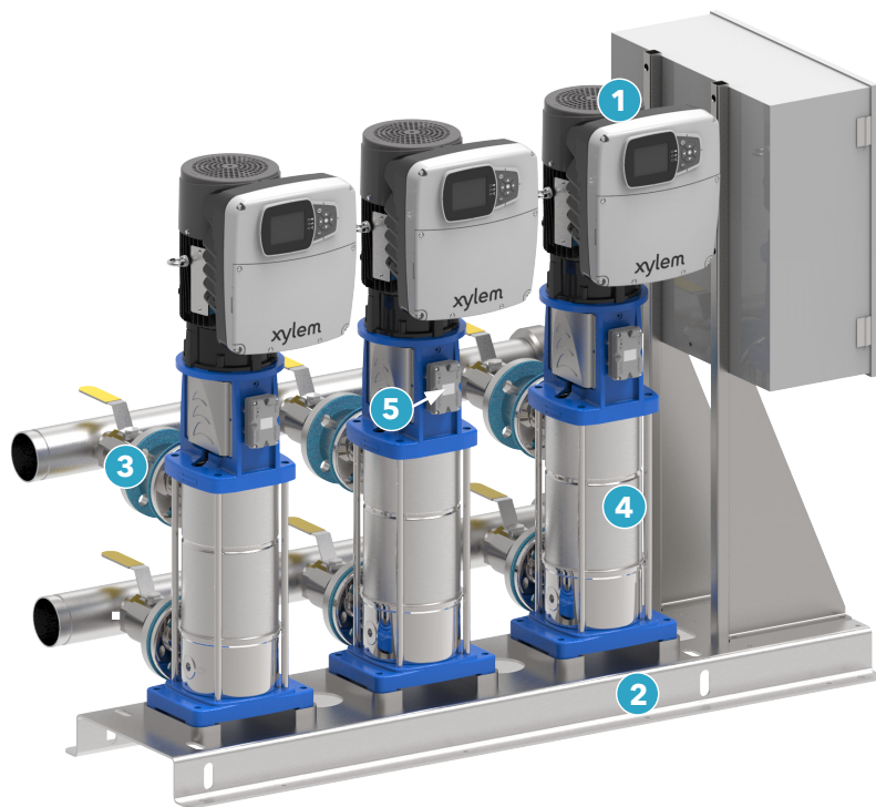
Système de poussée emballé TECHNOFORCE e-HVXR
