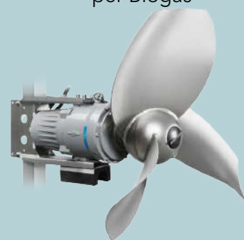
Mixer sommergibili per Biogas
